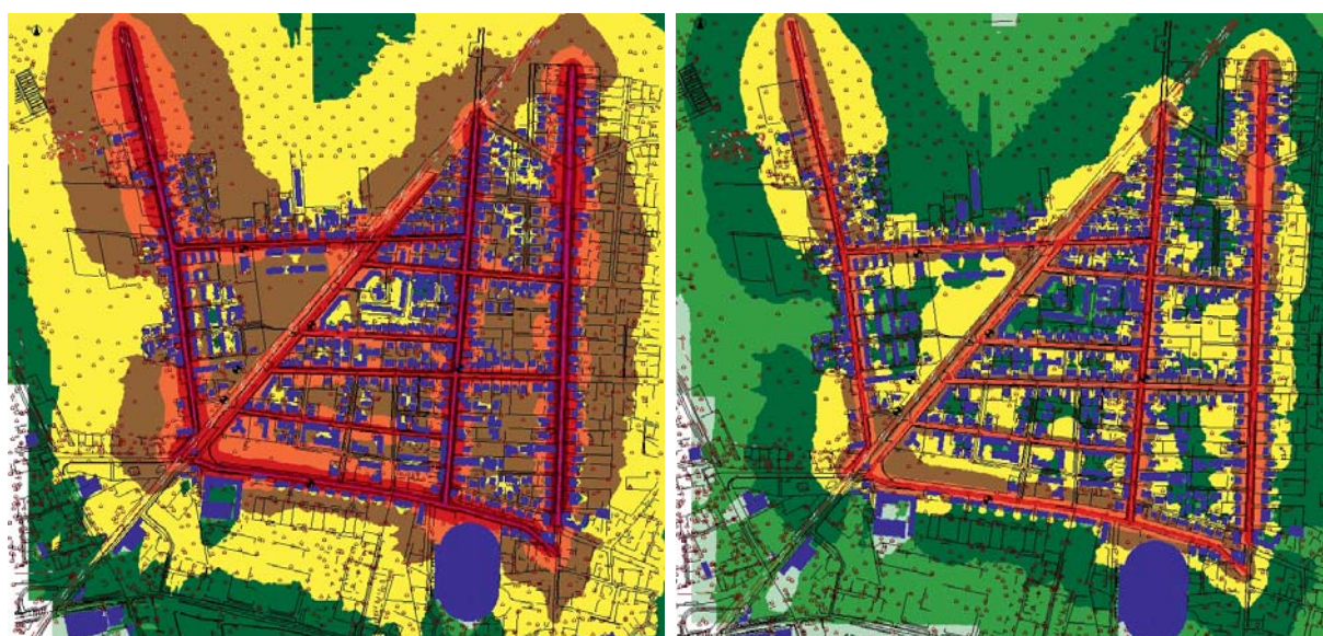
Figura A.1: Mapping in diurno (figura a sinistra) ed in notturno (figura a destra), relativi all'esposizione al solo rumore da traffico stradale, alla quota di 2 m.
