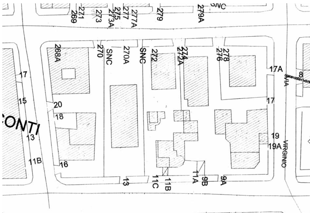
Figura n. 13.1.a: Esempio di edifici con distacco dalla sede stradale e con numero civico riferito al marciapiede
