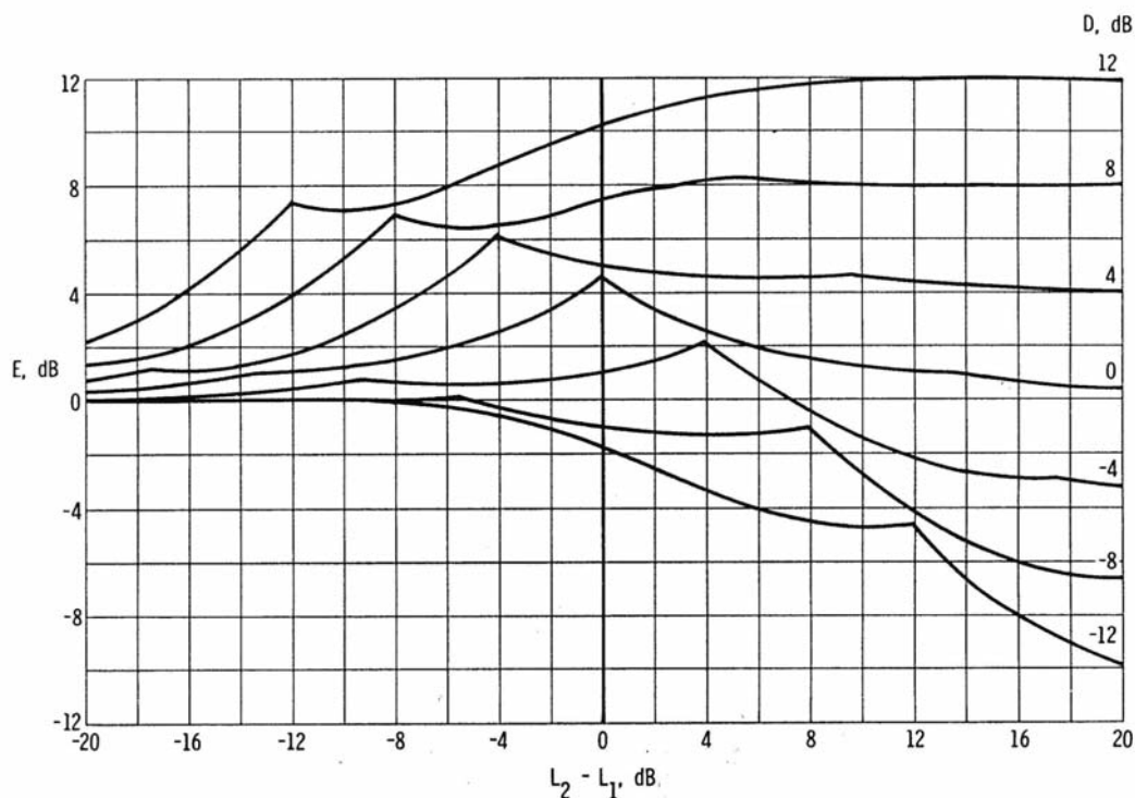
Figura. 10.2: Grafico proposto da Powell per la determinazione di E
