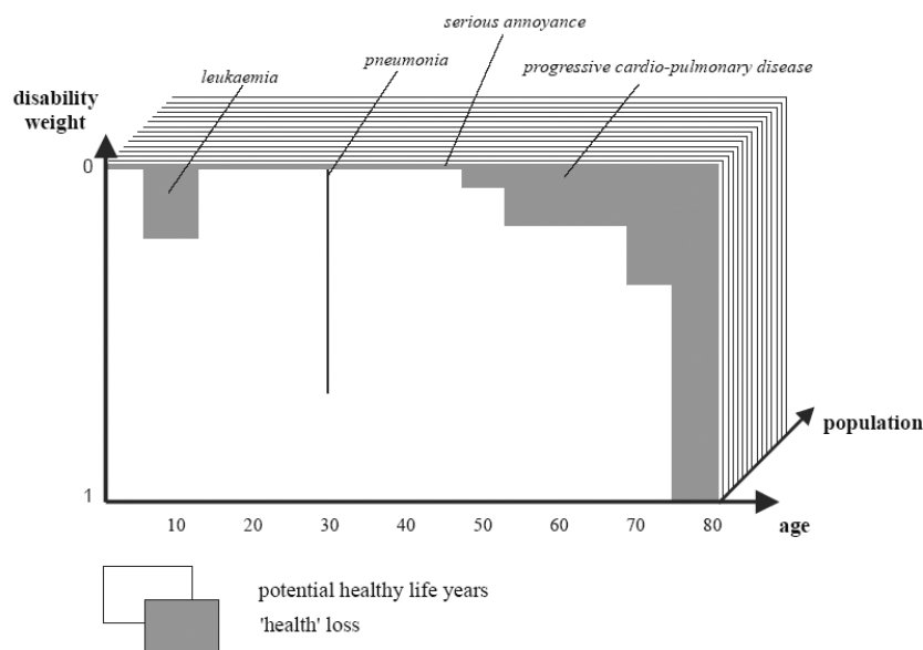
Figura 8.2: Diagramma esplicativo del concetto di DALY (Hollander et al. 1999).
