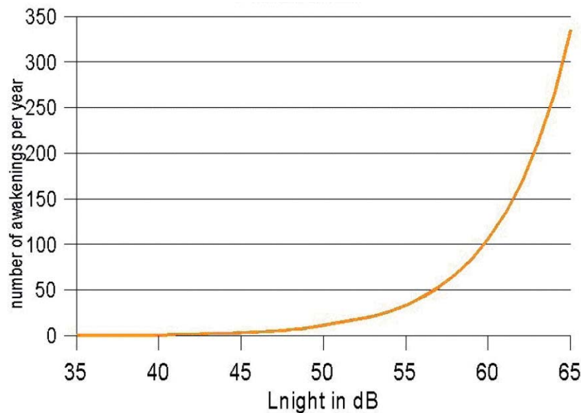
Figura 6.4: Numero di risvegli annui previsti in funzione del valore dell'indice acustico L_{night} in esterno. La figura illustra i risultati di un approccio di tipo cautelativo, riportando il numero massimo di risvegli atteso a tale livello di esposizione notturna.
