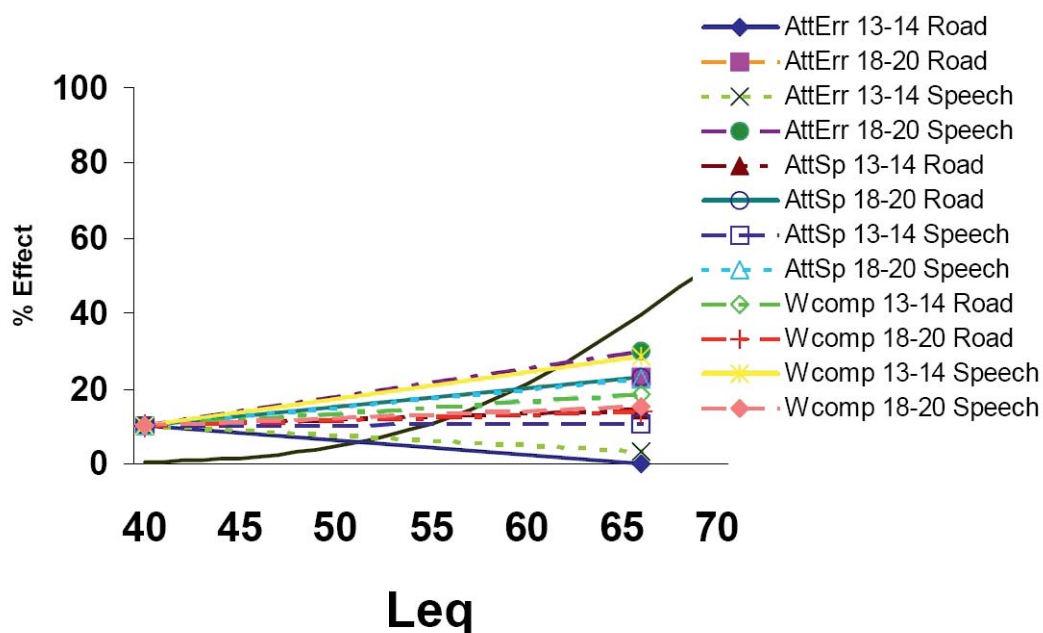
Figura 6.7: Curve dose-effetto e risultati da test svolti su bambini (13-14 anni) e giovani adulti (18-20 anni) esposti a rumore da traffico stradale o a rumore dovuto a conversazione a livelli di riferimento di 66 dB L_{eq} . AttErr = errori d'attenzione, AttSp = velocità di apprendimento, WComp = errori di comprensione verbale di un testo.
