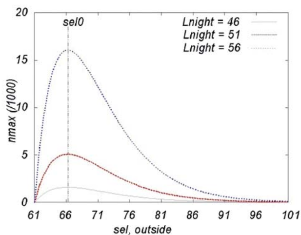
Figura 6.3: Valore massimo assunto da m/1000 per tre diversi valori di L_{night} all'interno della camera da letto dell'esposto e valori di SEL di eventi registrati invece in esterno.
