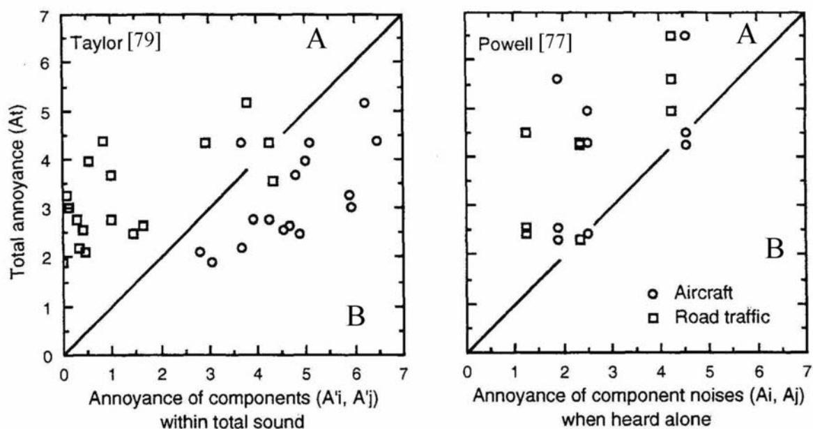
Figura 10.5: Confronto tra dati di multiesposizione raccolti in campo ed acquisiti in esperimenti in laboratorio
