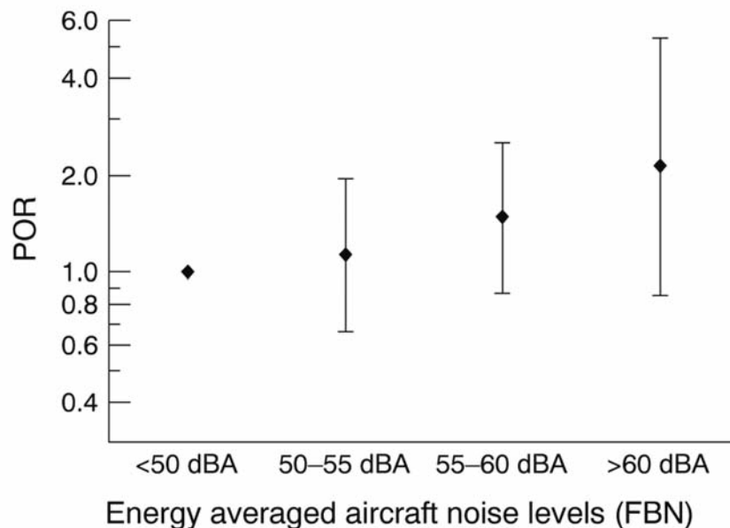
Figura 6.6: Rischio di ipertensione per esposizione a diverse classi acustiche di rumore aereo. I punti medi tra le barre indicano i valori corretti di odd ratio di prevalenza, le barre d'errore il 95% di intervallo di confidenza. (Rosenlund M., Berglind N., Pershagen G. et al., 2001)
