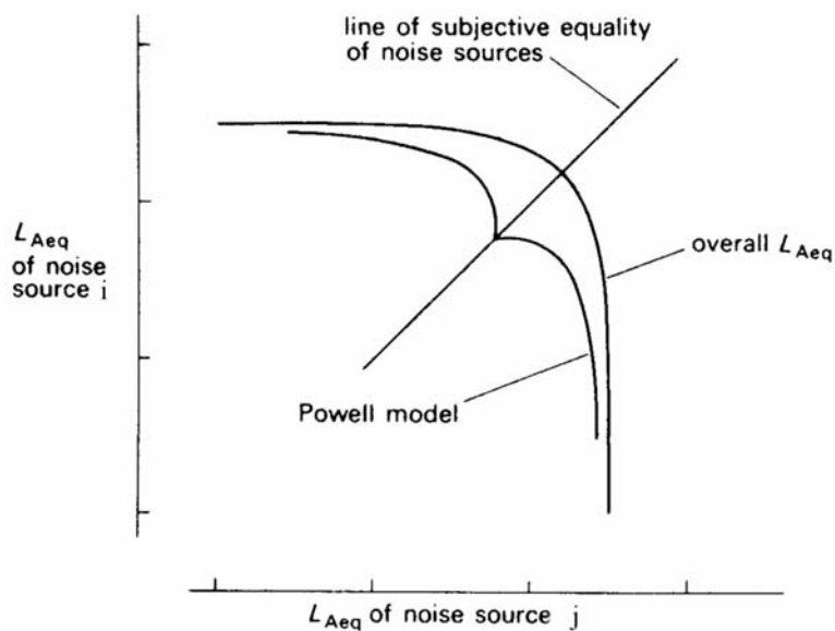
Figura 10.4: Rappresentazione del modello di Powell
