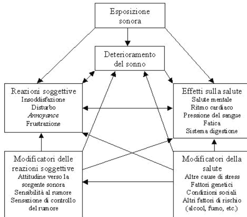
Figura: 4.1: Schema delle relazioni tra esposizione sonora, reazioni soggettive ed effetti sulla salute (Job, 1995).
