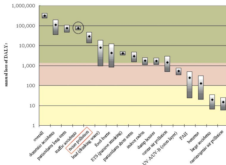
Figura 8.1: Istogramma del valore di DALY corrispondente a diverse cause di deterioramento della qualità della vita.
