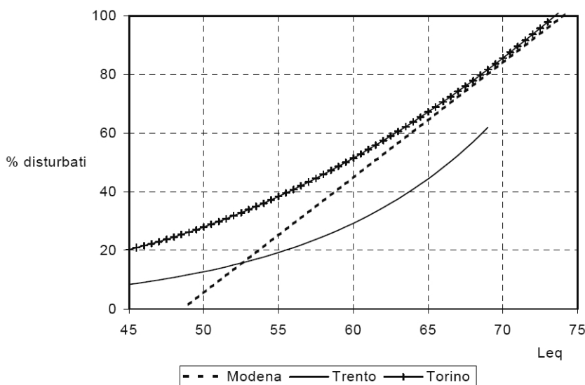
Figura 12: Percentuale di altamente disturbati in funzione del livello di esposizione notturno L_{eqA}(22-6)
