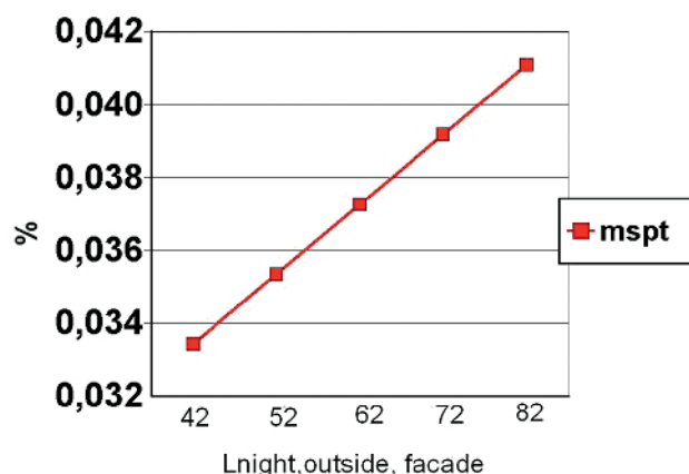
Figura 6.5: Crescita percentuale della motilità notturna media in funzione di L_{night, outside} .
