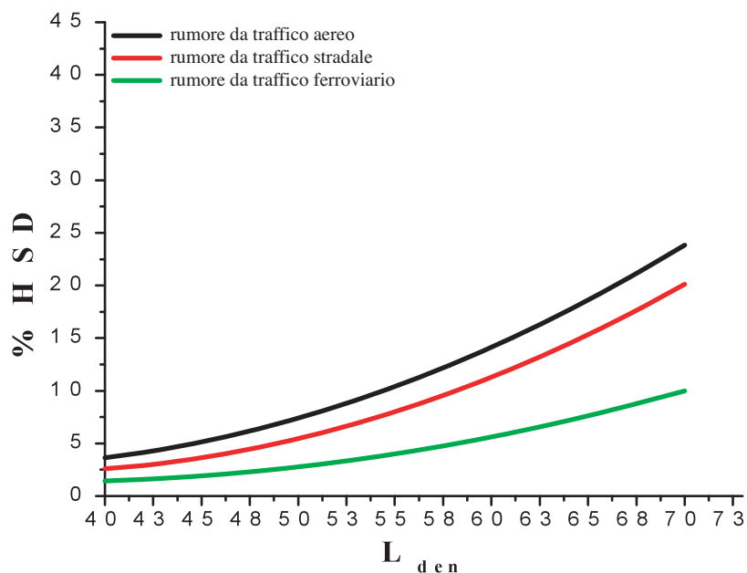
Figura 7.2: Percentuale di popolazione altamente disturbata da rumore in periodo notturno per esposizione a traffico aereo, stradale, o ferroviario.
