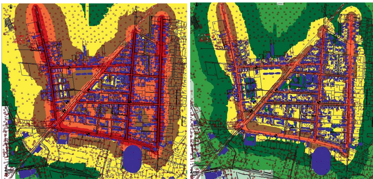
Figura A.3: Mapping in diurno (figura a sinistra) ed in notturno (figura a destra), relativi all'esposizione al solo rumore da traffico stradale, alla quota di 7.5 m.
