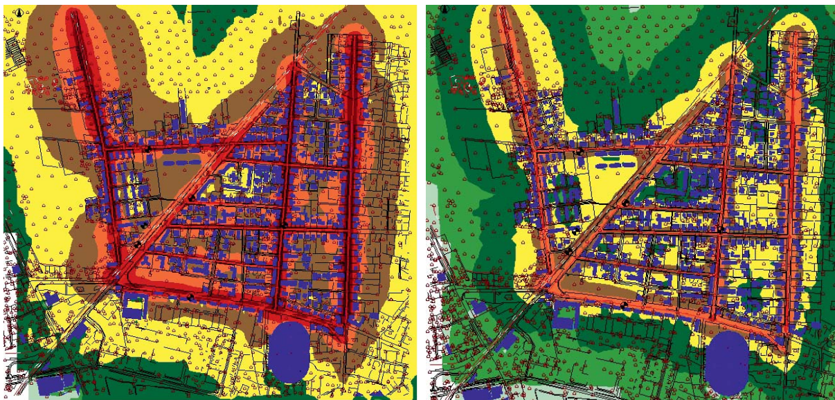
Figura A.2: Mapping in diurno (figura a sinistra) ed in notturno (figura a destra), relativi all'esposizione al solo rumore da traffico stradale, alla quota di 4 m.
