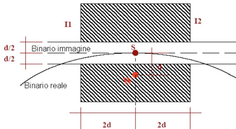
Figura 11.6.a: Suddivisione dell'area d'indagine in settori omogenei
