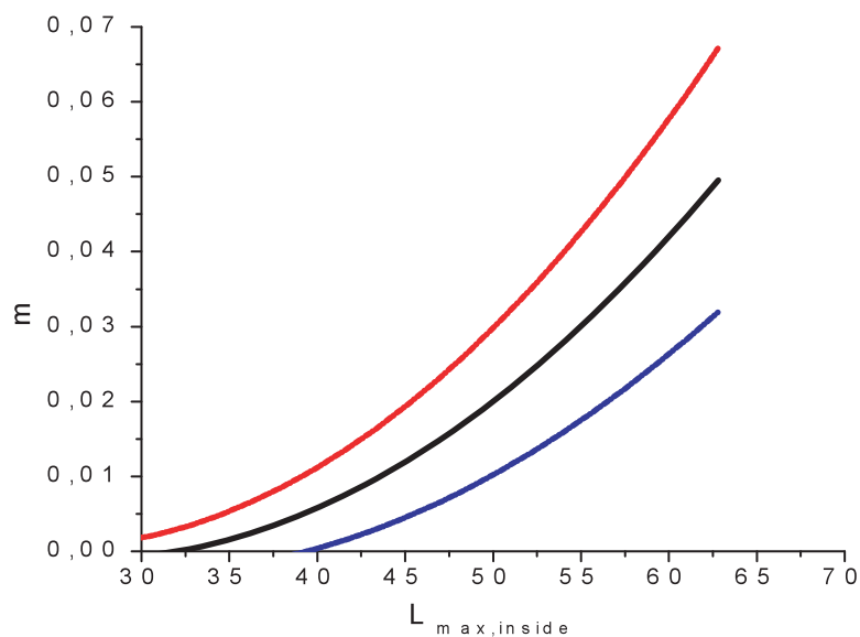
Figura 6.2: Andamento della probabilità di un incremento di motilità in funzione del valore di livello di immissione massimo in interno, contornato dalle linee dell'intervallo di confidenza al 95%. (Passchier-Vermeer et al., 2002).
