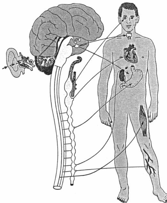
Figura: 5.1: Schema generale degli effetti extrauditivi dovuti all'esposizione sonora.
