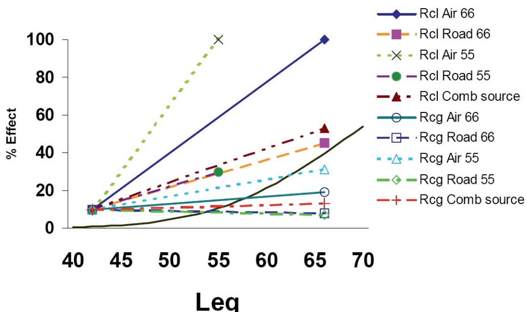
Figura 6.8: Curve dose-effetto e risultati da test svolti su bambini (13-14 anni) esposti a rumore da traffico di diversa tipologia e livello . Rcl = ricordo di un testo di recente lettura, Rcg = riconoscimento di un testo. Combsource = media dei diverse condizioni di esposizione derivanti da diverse sorgenti, con valori di immissioni di riferimento di 55 e 66 dB A di L_{eq}
