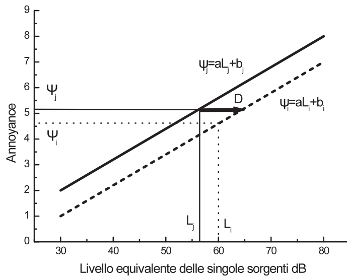
Figura 10.3: Ipotesi alla base del modello di Powell e significato del parametro D
