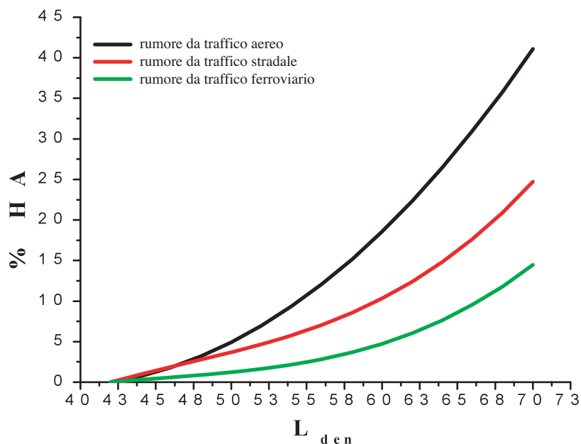
Figura 7.1: Percentuale di popolazione altamente disturbata da rumore in funzione di L_{den} per esposizione a traffico aereo, stradale, o ferroviario.
