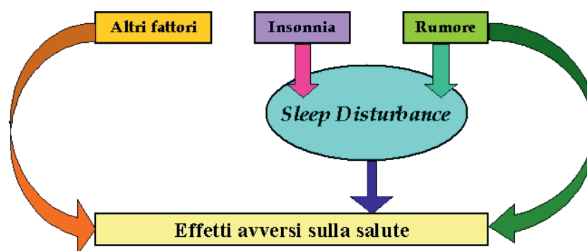
Figura 3.2.1: Possibile schema a blocchi sulle implicazioni fra rumore e salute.
