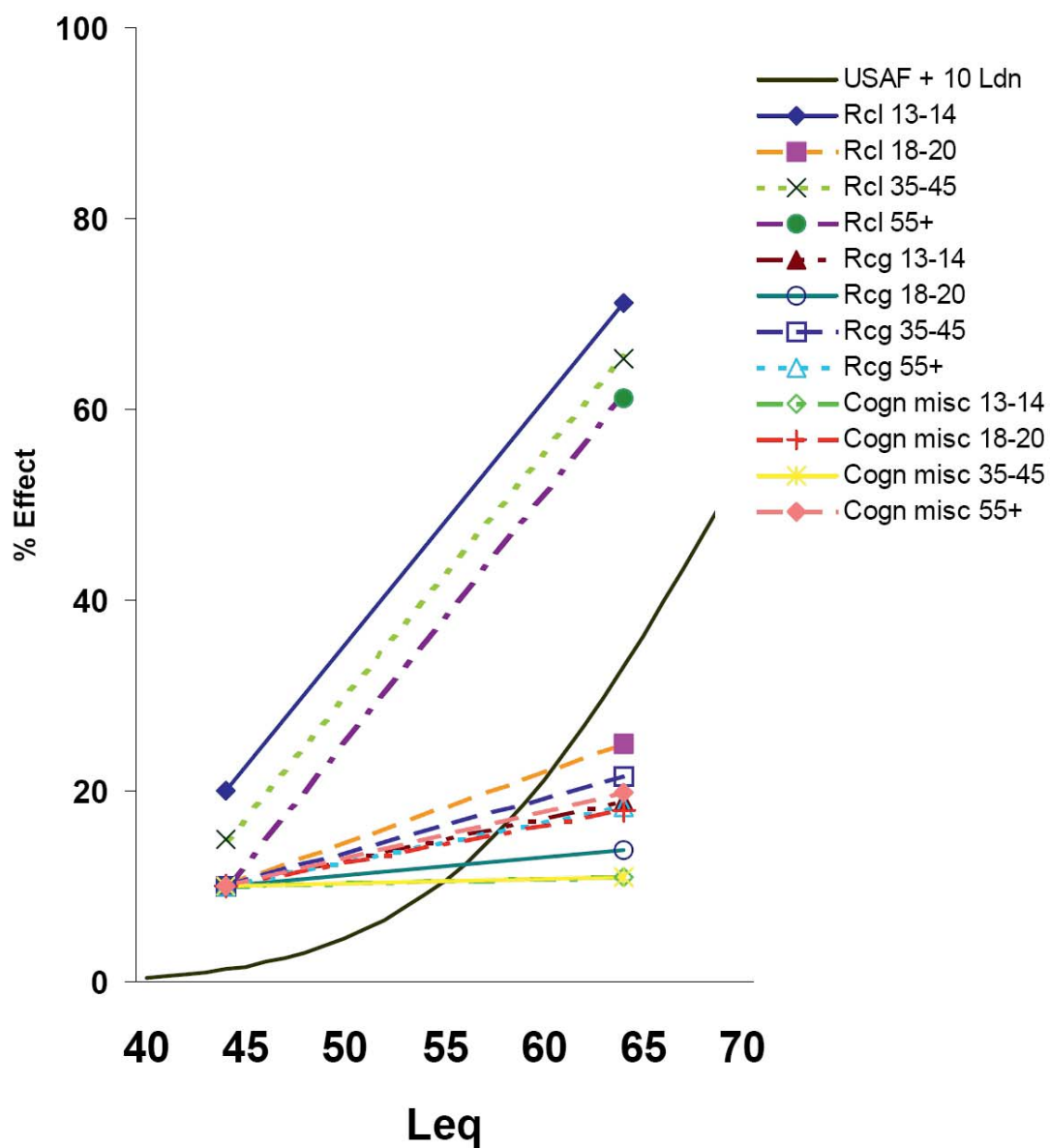
Figura 6.9: Curve dose-effetto e risultati di test svolti su adolescenti (13-14 anni), giovani adulti (18-20 anni) e persone di mezza età (35-45 anni) esposti a rumore da traffico stradale o a rumore dovuto a conversazione, a livelli di riferimento di 66 dB L_{eq} . Rcl = ricordo di un testo di recente lettura, Rcg = riconoscimento di un testo, Cogn misc = valor medio dei risultati derivanti da altri esperimenti sull'attenzione e la comprensione delle parole.
