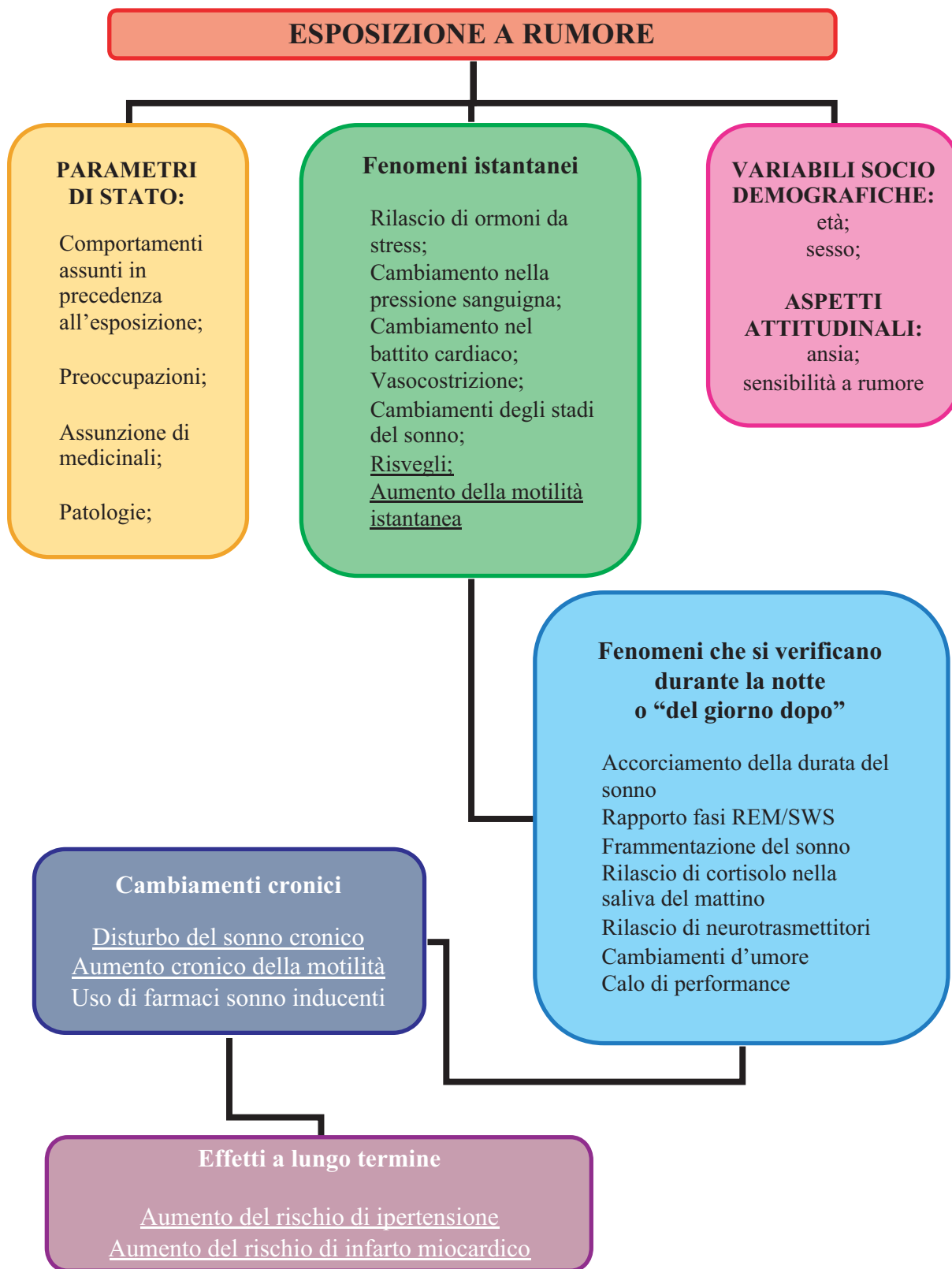
Figura 6.1: Diagramma degli effetti specifici coinvolti nel disturbo del sonno prodotto dal rumore ambientale (Ising, 1999).
