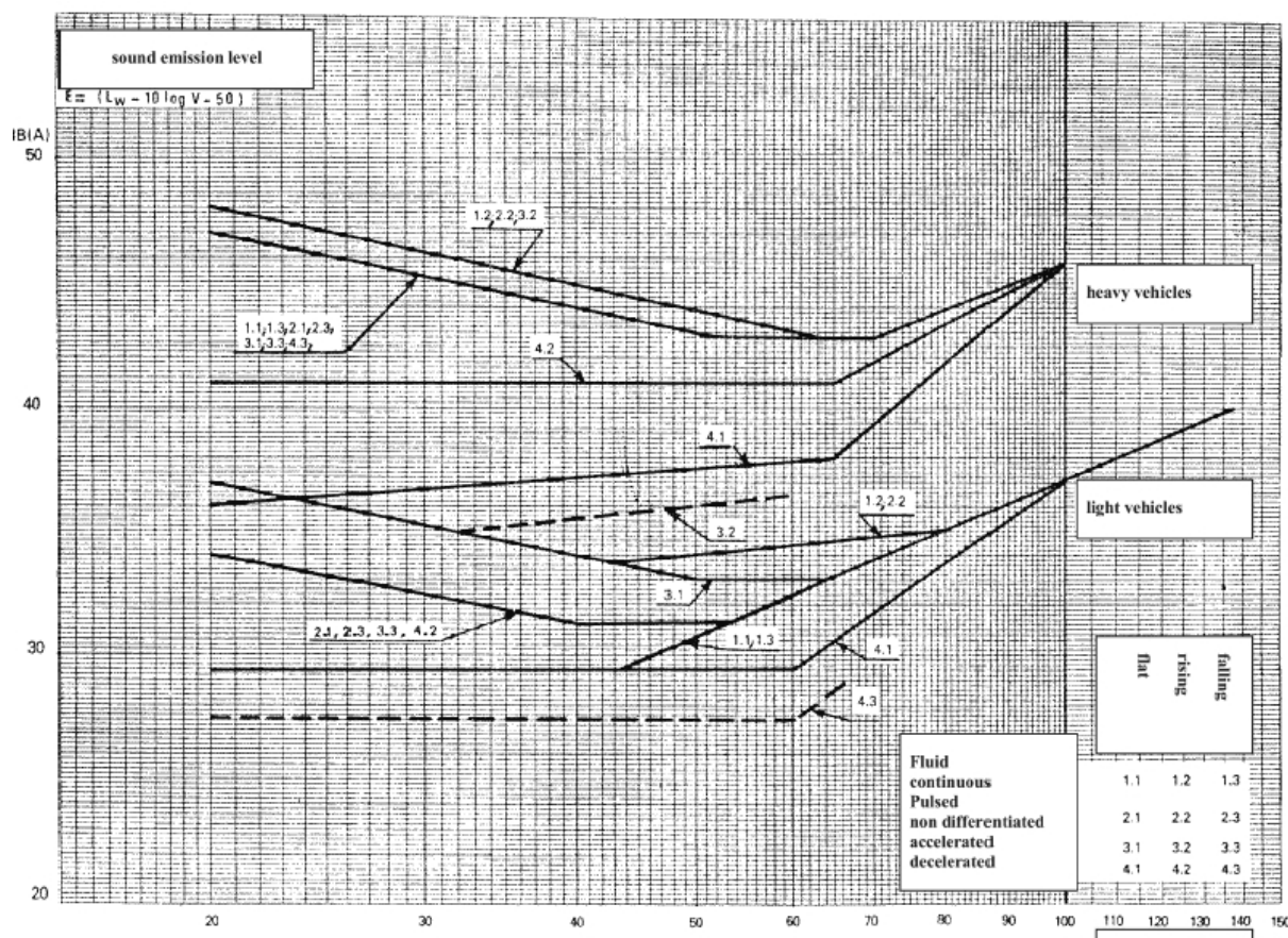
Figura n. 11.7.1: Emissione sonora del singolo veicolo ( L_{Aeq,h} ) per varie condizioni di marcia.
