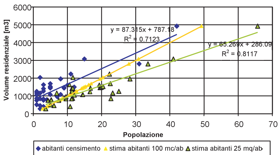
Figura n. 13.2.c: Stima della popolazione mediante indici indiretti volumetrici e areali.
