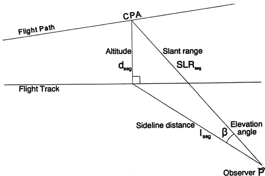
Figura 11.8.2: Costruzione della traiettoria tridimensionale di volo (flight path)
