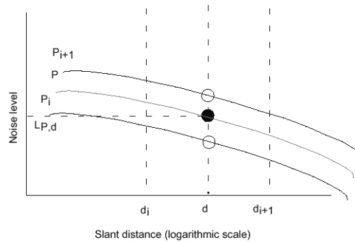
Figura 11.8.3: Determinazione del valore L_{Pd} da valori noti di potenza e slant distance.
